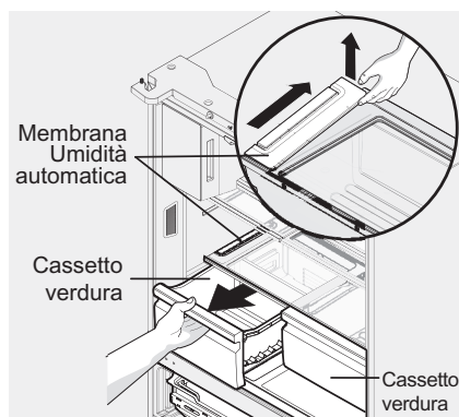
Rimozione membrana controllo automatico umidità
