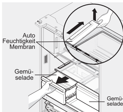
Ausschalten der Auto-Feuchtigkeit Kontrolle der Membran
