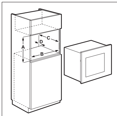
Asennuksen vähimmäisetäisyydet
