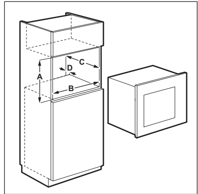
Monteringsavstånd
